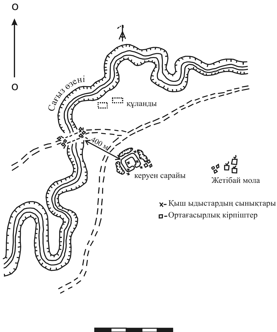
2-сур. Таскешу көпірі құландысының схемалық планы [10]
