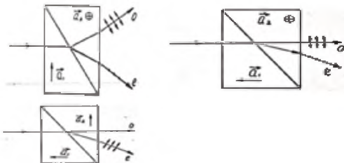
Сурет 1 – а) Волластон призма; б) Рошон призмасы; в) Сенармон призмасы.
