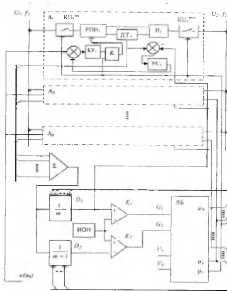
Рисунок 2 – Модульная преобразовательная система с варьированием числа агрегатов в зависимости от величины и характера нагрузки.
