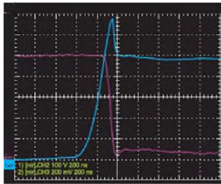
Рисунок 2 – Для «короткого» контура модуля: а) распределенная паразитная индуктивность; б) переходный процесс коммутации ( I_k - 20 А/дел; U_{кз} - 100 В/дел; t - 200 нс/дел)
