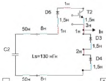
Рисунок 2 – Для «короткого» контура модуля: а) распределенная паразитная индуктивность; б) переходный процесс коммутации ( I_k - 20 А/дел; U_{кз} - 100 В/дел; t - 200 нс/дел)
