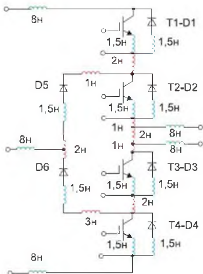
Рисунок 1 – Эквивалентная схема модуля инвертора с паразитными индуктивностями
