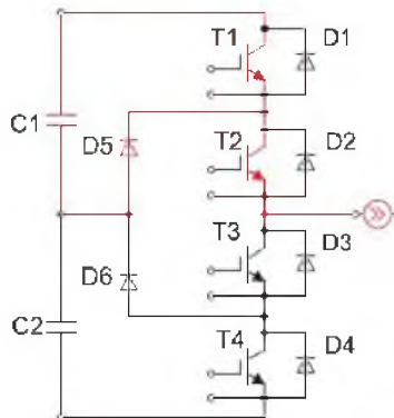
Рисунок 2 – Первый контур коммутации
