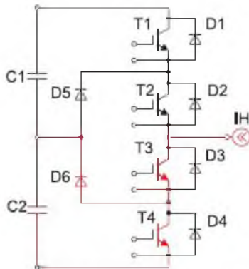
Рисунок 4 – Третий контур коммутации
