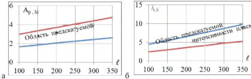
Рисунок 3 – Верхняя и нижняя границы предсказуемой интенсивности однополувольтной пляски. а) – для V_1 = 5 м/сек ; б) - для V_1 = 15 м/сек ;
