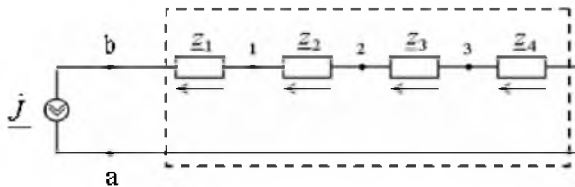
Рисунок 2 – Незвращенная цепь
