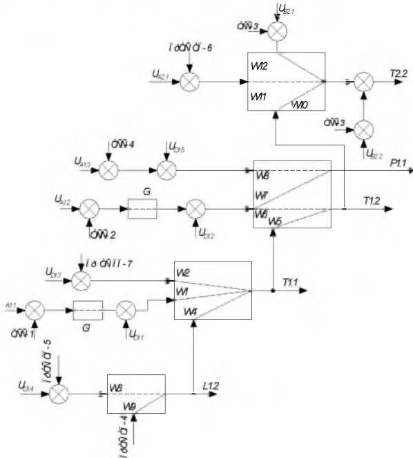
Рисунок 1 – Структурная схема воздухоподогревателя как объекта управления
