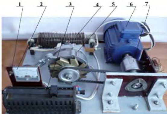
Рисунок 1 – Трехфазный АД, нагруженный на генератор:
