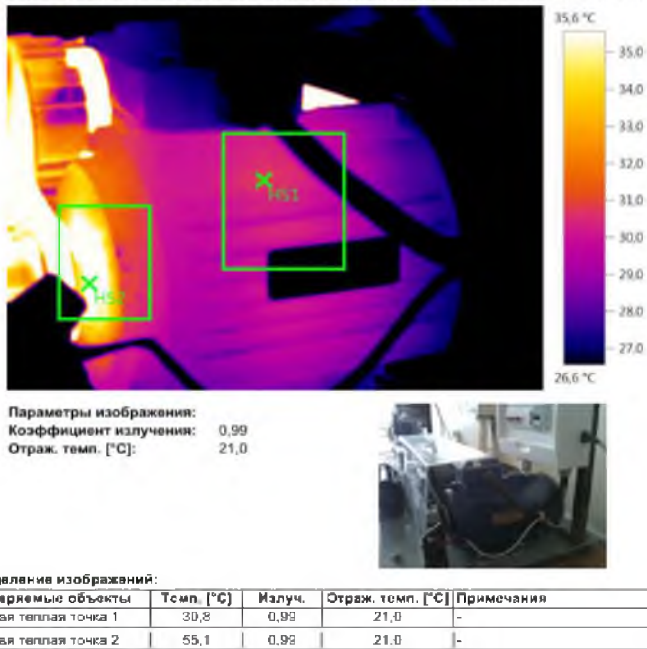
Рисунок – 4 Измерение температурного поля АД с применением тепловизора
