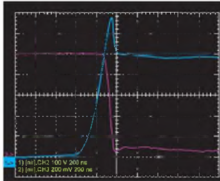
Рисунок 3 – Для «длинного» контура модуля инвертора: а) распределенная паразитная индуктивность; б) переходный процесс коммутации ( I_k - 20 А/дел; U_{кз} - 100 В/дел; t - 200 нс/дел)
