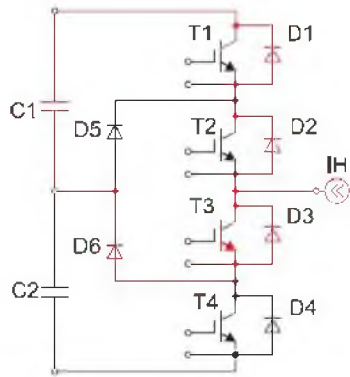
Рисунок 3 – Второй контур коммутации
