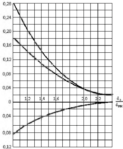
Рисунок 2 – Распределение напряженности магнитного поля вне индуктора при \frac{d_3}{d_{ИБ}} = 0,6 (расчетные): 1 – составляющая напряженности от тока индуктора; 2 – составляющая напряженности от токов в нагрузке; 3 – результирующая напряженность магнитного поля
