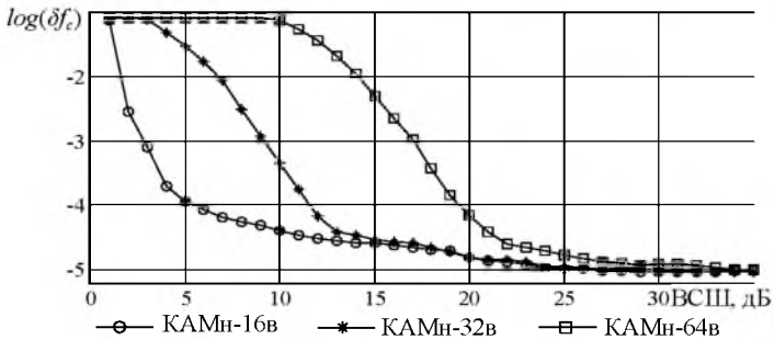
Рисунок 4 – Зависимости относительной ошибки определения несущей частоты КАМн сигналов от ОСШ
