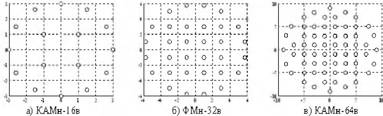
Рисунок 1 – Закругленные фазовые созвездия КАМн
