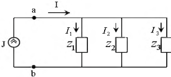
Рисунок 3 – Параллельная цепь
