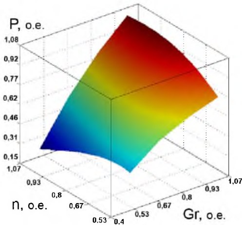
Рисунок 2 – Зависимость абсолютного расхода топлива Gr , оборотов двигателя n и развиваемой мощности P ДЭС
