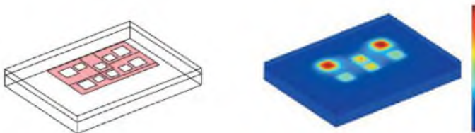
Рисунок 6 – Температурное поле в конструкции силового модуля инвертора: заметно нагреты транзисторы Т1 и Т4 по сравнению с транзисторами Т2 и Т3
