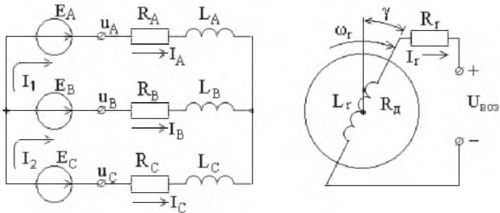
Рисунок 1 – Схема распределения токов в обмотках синхронного компенсатора
