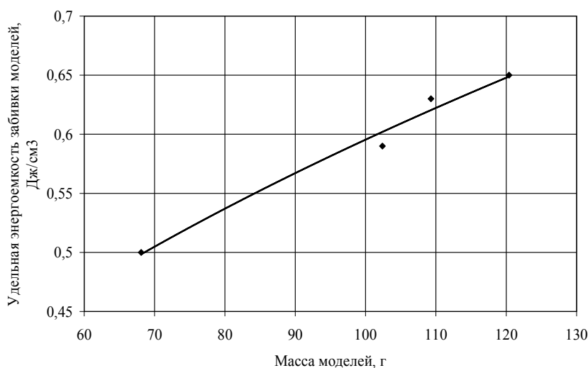
Рис. 6. Зависимость удельной энергоёмкости моделей свай от их массы
