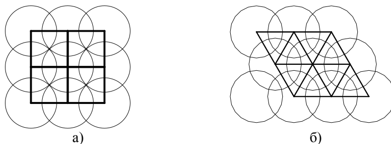
Рис. 3. Схемы размещения точек уплотнения грунта трамбовками по вершинам квадрата (а), равностороннего треугольника (б)
