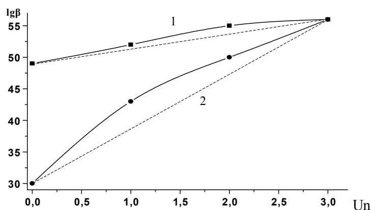
Рис. 1. Зависимость констант образования смешаннолигандных комплексов от числа координированных групп унитиола
