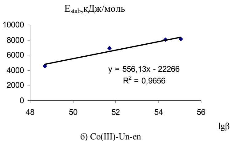
Рис 2. Зависимости E_{\text{stab}} от констант устойчивости
