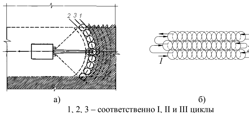
Рис. 2. Схема уплотнения грунтовых оснований с перекрытием следов: а) трехцикловая (по два-три удара в каждом цикле с повторением циклов до получения отказа); б) двухцикловая (по пять-шесть ударов в цикле).
