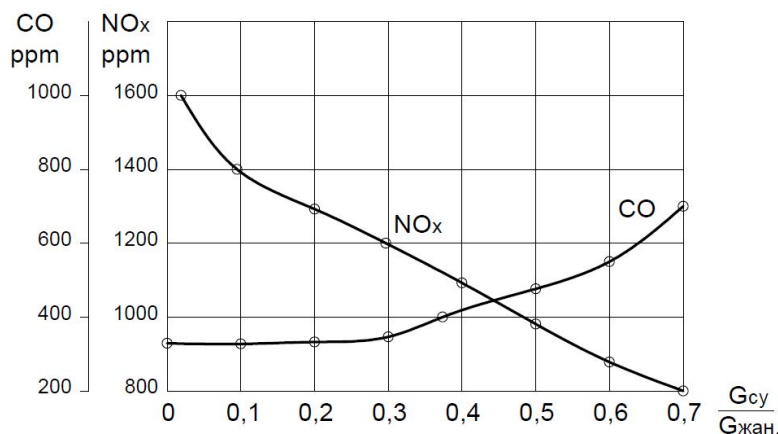
Сурет 1. Абтхоф пен Лютер [1] зерттеулері бойынша жанғыш қоспаға бүркілген су мөлшеріне байланысты шығынды газдар құрамындағы улы заттардың ( \text{NO}_x пен \text{CO} ) өзгеруі
