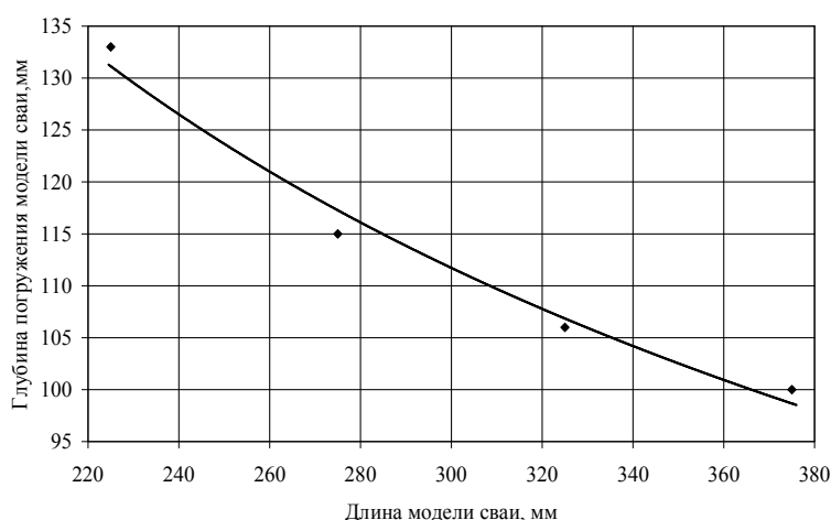
Рис. 3. Зависимость глубины погружения моделей свай от их длины
