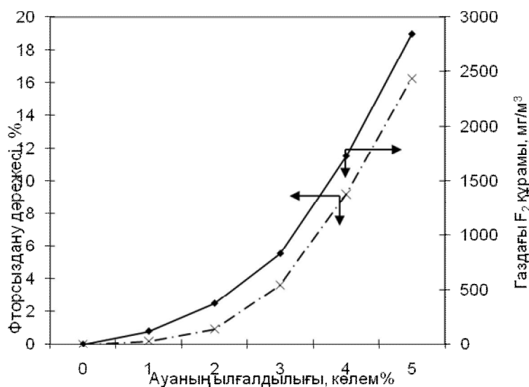
Сурет 3. Газдағы F 2 концентрациясына байланысты және шихтаның пісіру қабатына түсетін ауадағы H 2 O буынның құрамындағы фтордың жойылу дәрежесі
