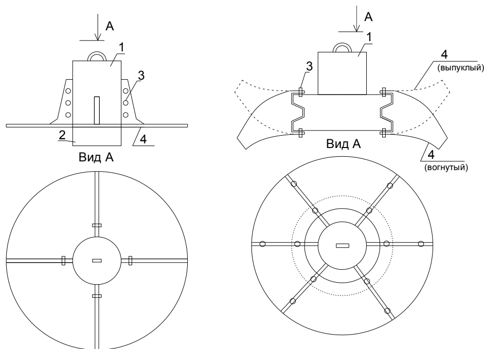
Рис. 8. Конструктивная схема тяжёлых трамбовок: а) рекомендуемая по ТКП [6]; б) предлагаемая авторами.
