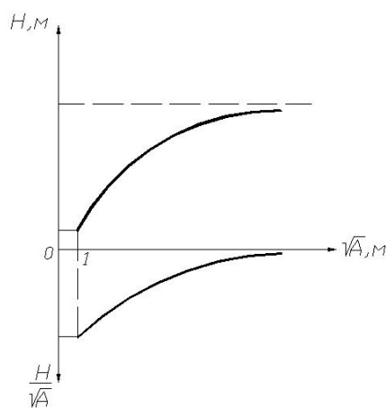
Рис. 1. Предполагаемые зависимости глубины сжимаемой толщи H и соотношения \frac{H}{\sqrt{A}} от размеров фундамента \sqrt{A} (при d=\text{const} ; p=\text{const} )
