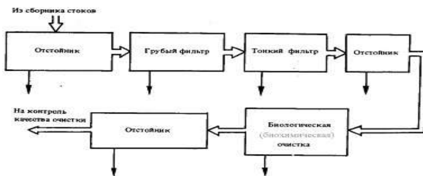
Рис.8. Принципиальная схема очистки сточных вод
