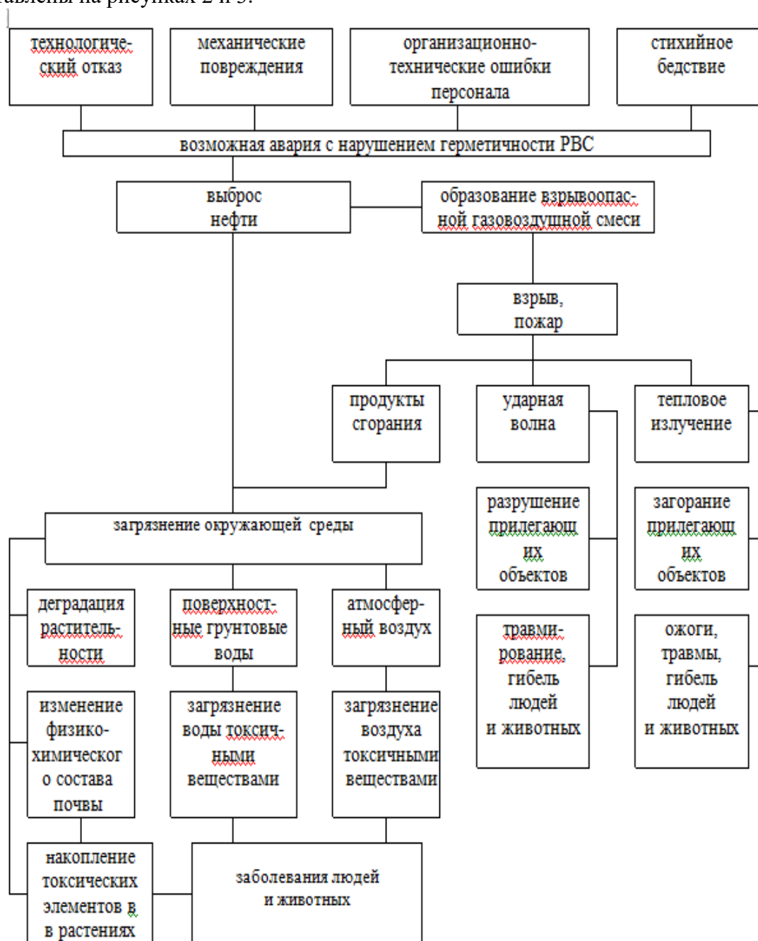
Рисунок 2. Блок-схема вероятного развития аварии при разгерметизации РВС.
