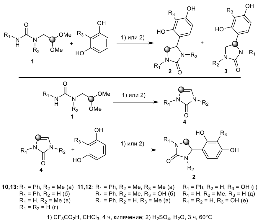
Схема 3 - Взаимодействие фенолов с α-уреидоацетальями
