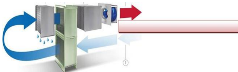
Сурет 3 – Қауынды кептіру желісіндегі ауа қозғалысы
