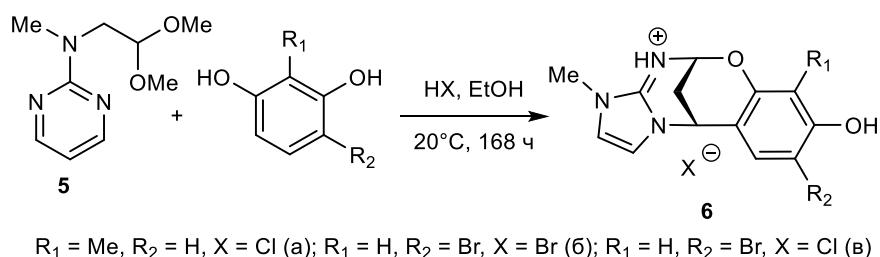
Схема 4 - Взаимодействие фенолов с пиридинсодержащим ацеталем
