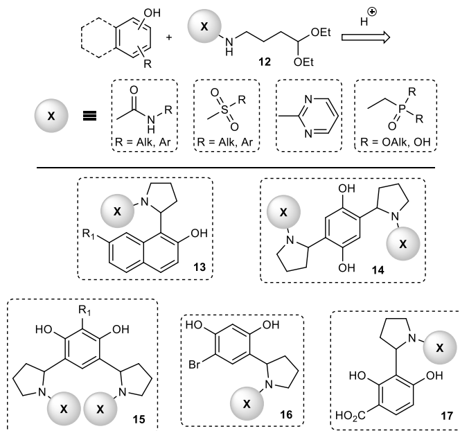
Схема 8 - Взаимодействие фенолов с \gamma -функционализированными ацетальми
