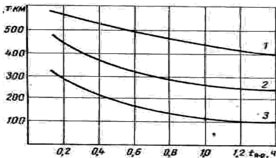
Рисунок 1 - График изменение производительности автомобилей в зависимости от времени простоя под погрузкой-разгрузкой
