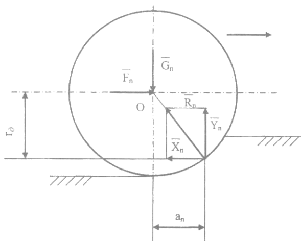
Рисунок 1 - Силы, действующие на ведомое колесо
