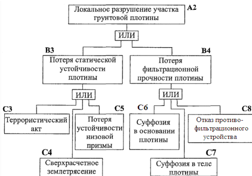
Рисунок 4 - «Дерево отказов» для сценария аварии A2
