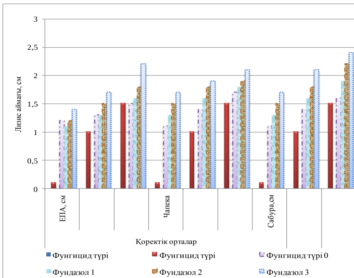
Сурет 5 - Фундазолдың топырақ микробоценозына әсері
