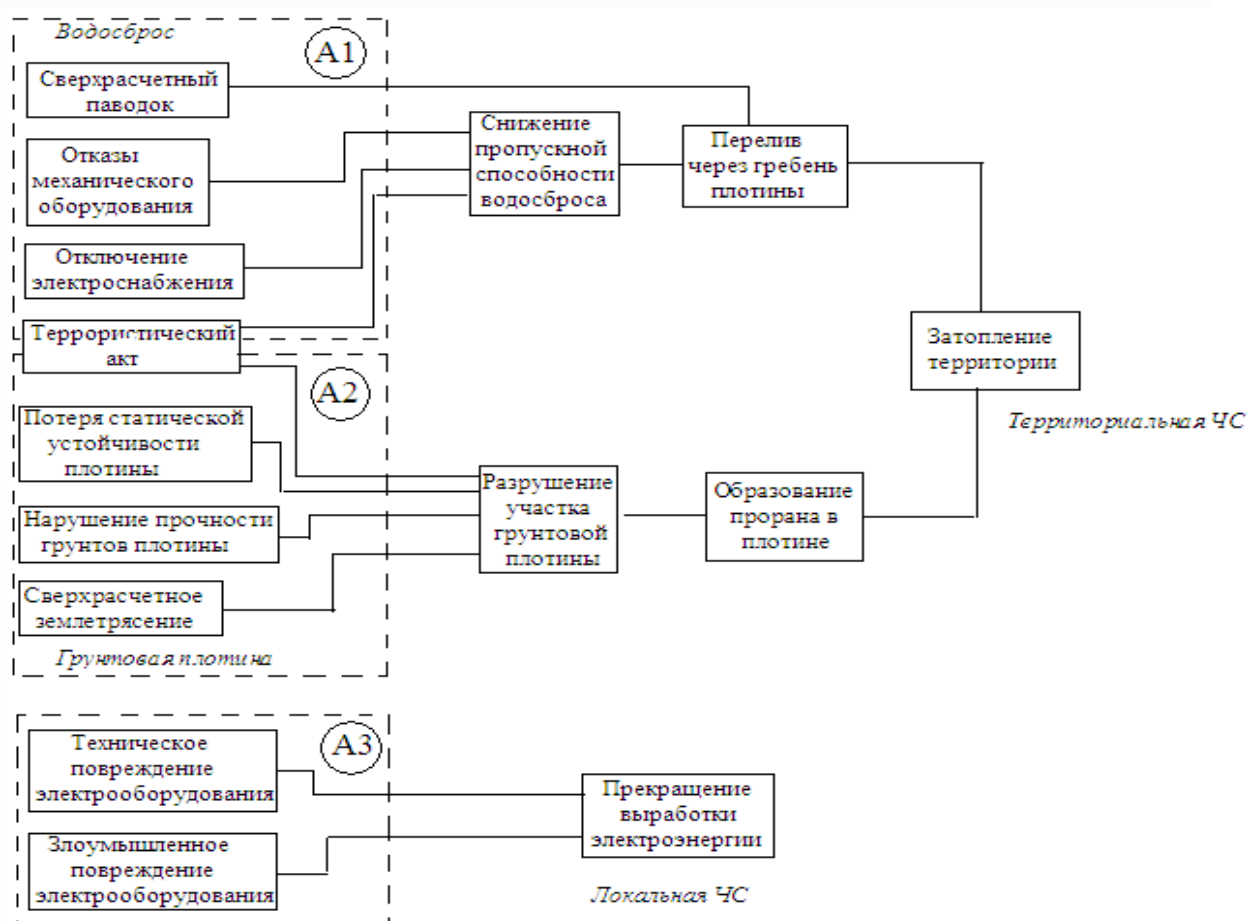
Рисунок 2 – Блок-схема анализа основных вероятных сценариев аварий на каскаде Алматинских ГЭС
