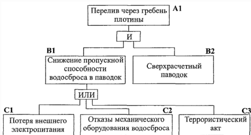
Рисунок 3 - «Дерево отказов» для сценария аварии А1
