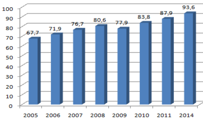
Диаграмма 2- Потребление электроэнергии в Казахстане по годам (млрд кВт ч) [2]
