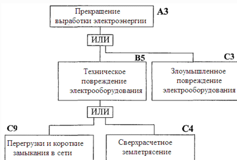
Рисунок 5 - «Дерево отказов» для сценария аварии A3
