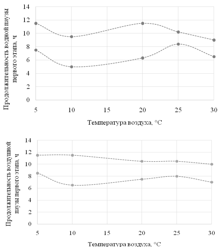
Рис. 4. График для определения оптимальной продолжительности водной и воздушной пауз процесса проращивания зерна пшеницы
