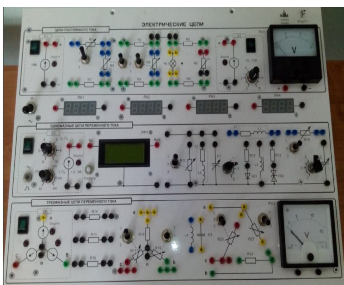
Сурет. «Электрлік тізбесі кешені» байланыс алаңшаларынан тұратын қондырғы
