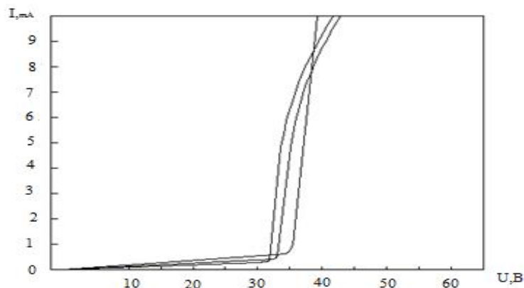
Рис. 1. Вольт-амперные характеристика стабилизатора
