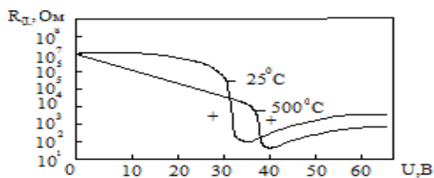
Рис. 2. Характеристики дифференциального сопротивления стабилизирующих структур в различных температурных режимах
